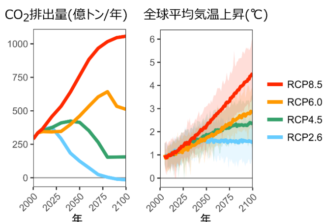
図 S2 : 各 RCP シナリオにおける CO2 排出量（左）と、それに基づいてシミュレーションされた全球平均気温上昇（右）。
